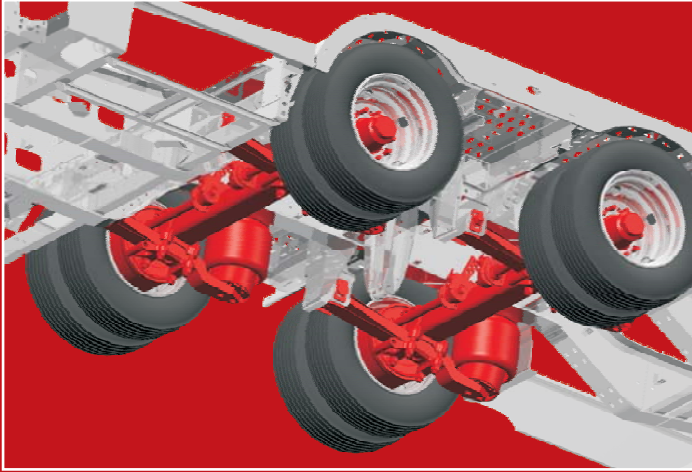
Zwillingsbereifung für hohe Nutzlast und Rollbälge für außergewöhnliche Fahrstabilität.
